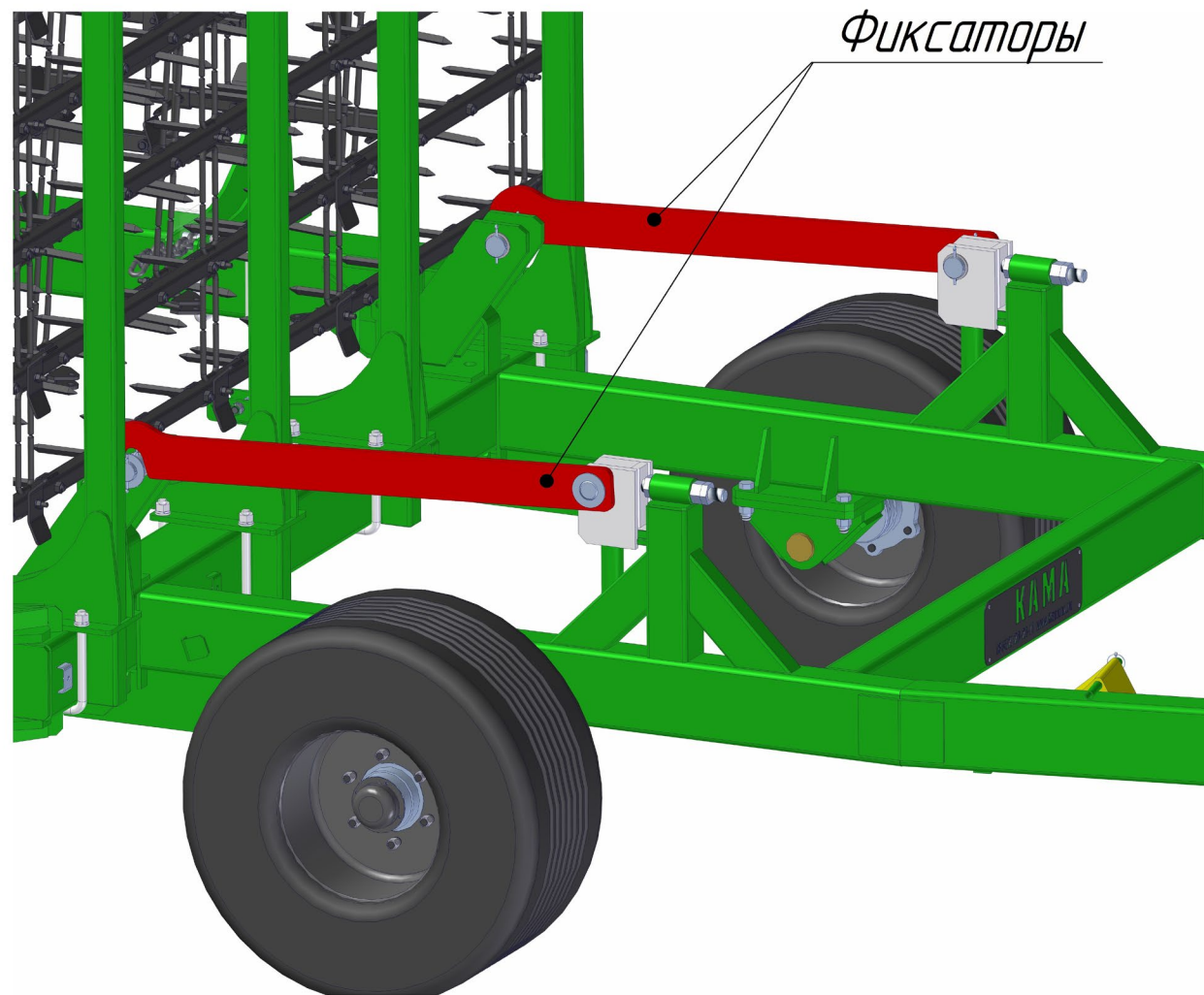
Рисунок 20 - Фиксаторы гидроцилиндров
