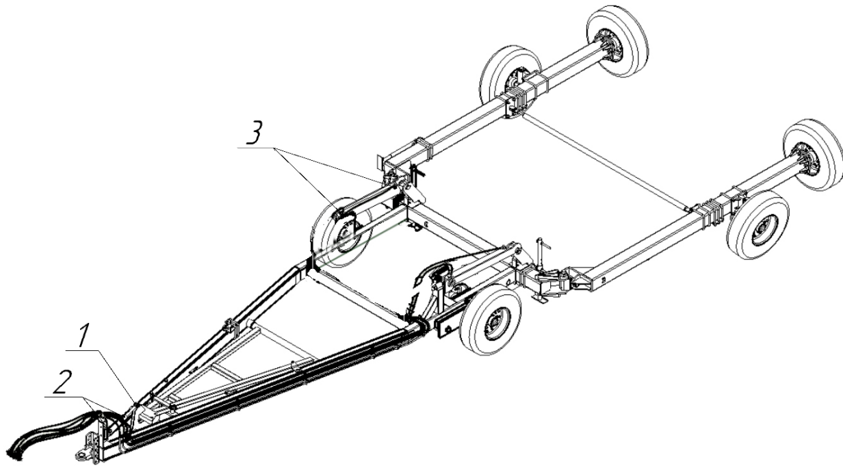
Рисунок 16 – Гидросистема
