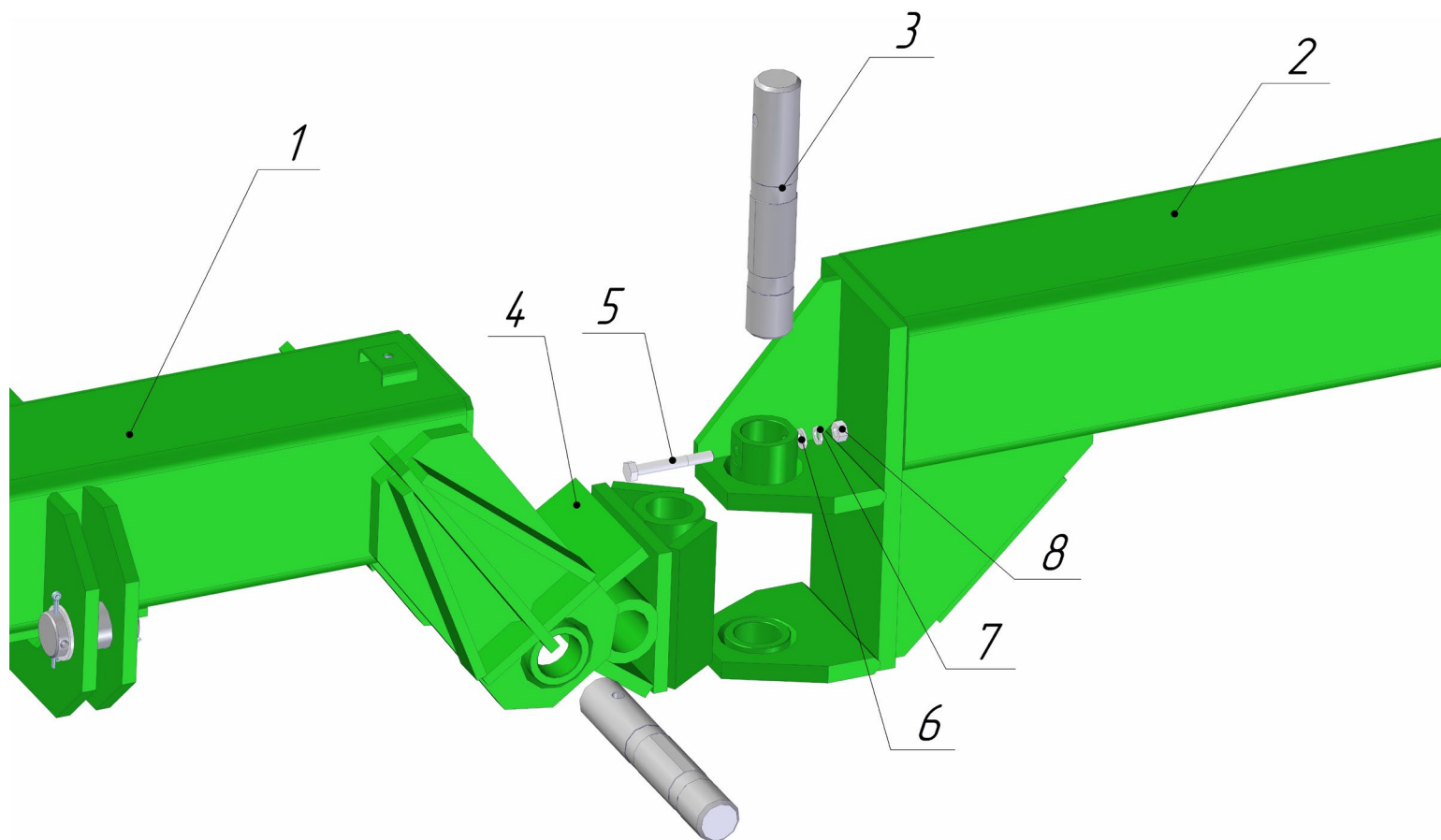
Рисунок 6- Установка балок поперечной и продольной
