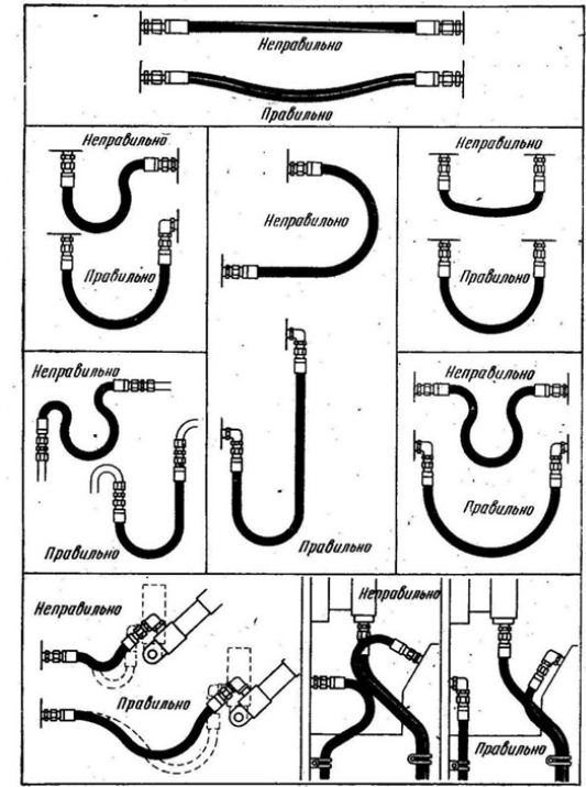
Рисунок 17 - Рекомендация по прокладке РВД
