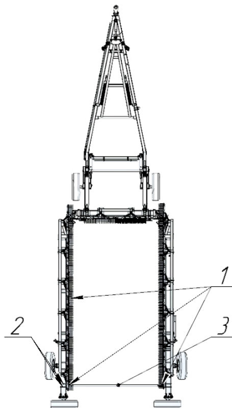
Рисунок 18 - Установка стяжки
